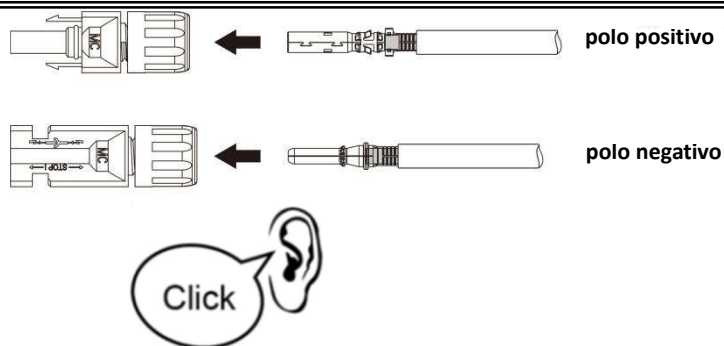
Figura 5-12 Conexão do cabo CC (3)
