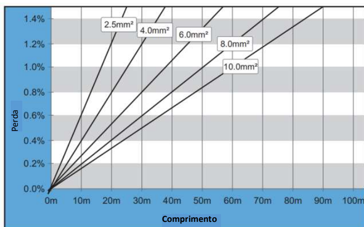
Figura 5-6 Relação entre comprimento, secção transversal e perda de potência do cabo
