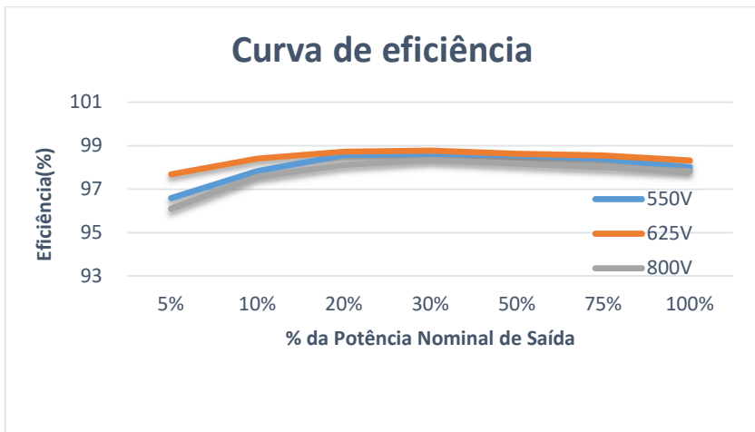
Figura 2-8 Curva de eficiência em potência (exemplo para 80kW)
