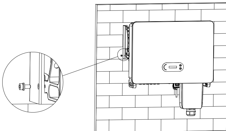
Figura 4-9 Fixe o inversor
