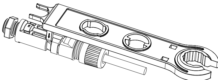
Figura 5-15 Remoção de conector CC
