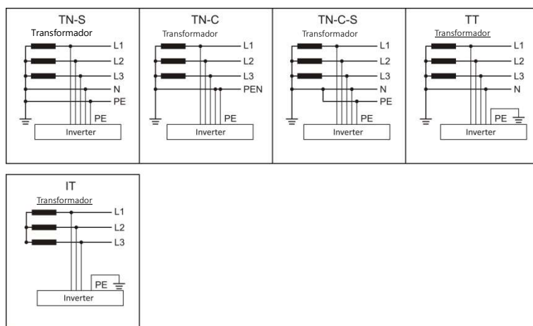
Figura2-2 Visão geral dos tipos de rede
