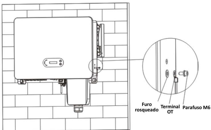
Figura 5-4 Diagrama de instruções para aterramento externo do inversor
