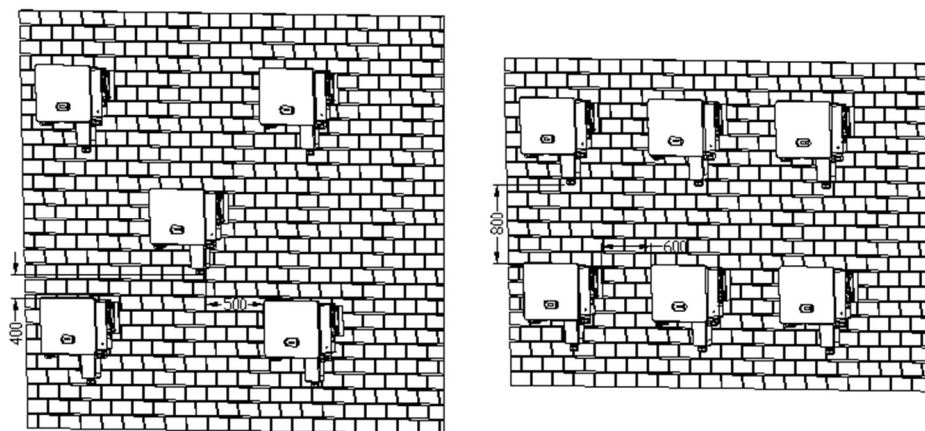
Figura 4-3 Espaçamentos para múltiplos inversores 60~80KTLX-G3
