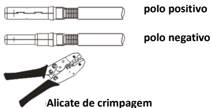
Figura 5-11 Conexão do cabo CC (2)
