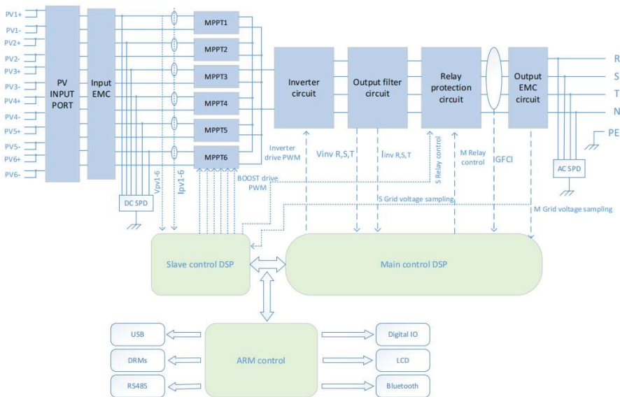
Figura 2-7 Estrutura do circuito principal
