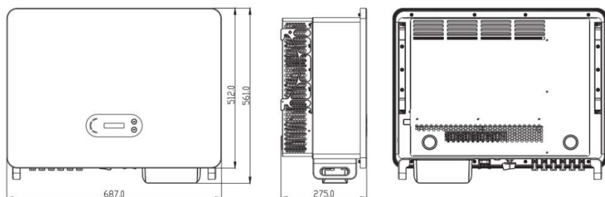
Figura 2-3 Frente, lado e traseira da máquina (80kW)
