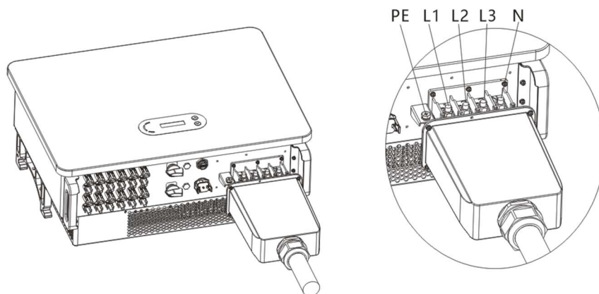
Figura 5-9 Diagrama de instruções de conexão do cabo CA (2)
