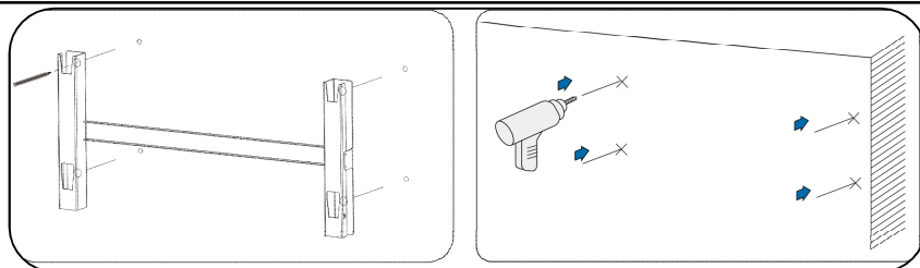
Figura 4-6 Fazendo as furações na parede de montagem
