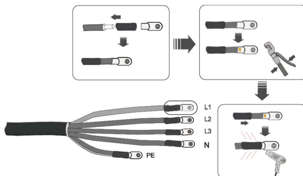
Figura 5-8 Diagrama de instruções para conexão de cabo CA (1)
