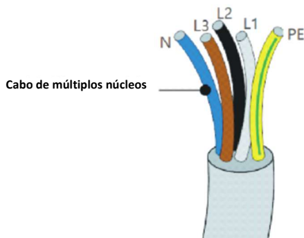
Figura 5-7 O cabo de múltiplos núcleos para o equipamento
