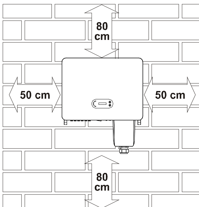
Figura 4-2 Espaços para inversor individual
