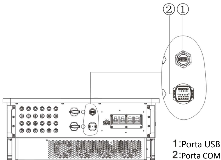
Figura 5-16 Porta de conexão de comunicação
