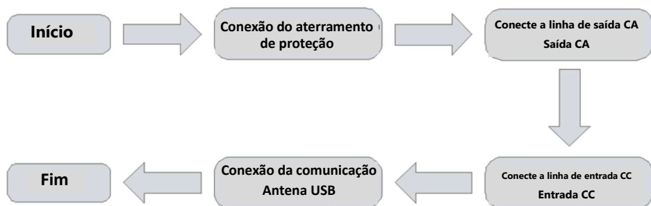
Figura 5-1 Fluxograma de conexão dos cabos ao inversor
