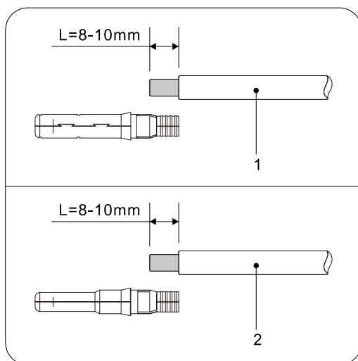
Figura 5-10 Conexão do cabo CC (1)
