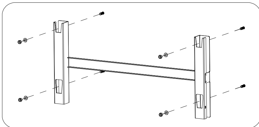
Figura 4-8 Instalação do painel traseiro
