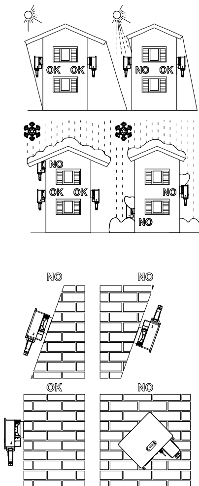
Figura 4-1 Escolha da Posição de Instalação
